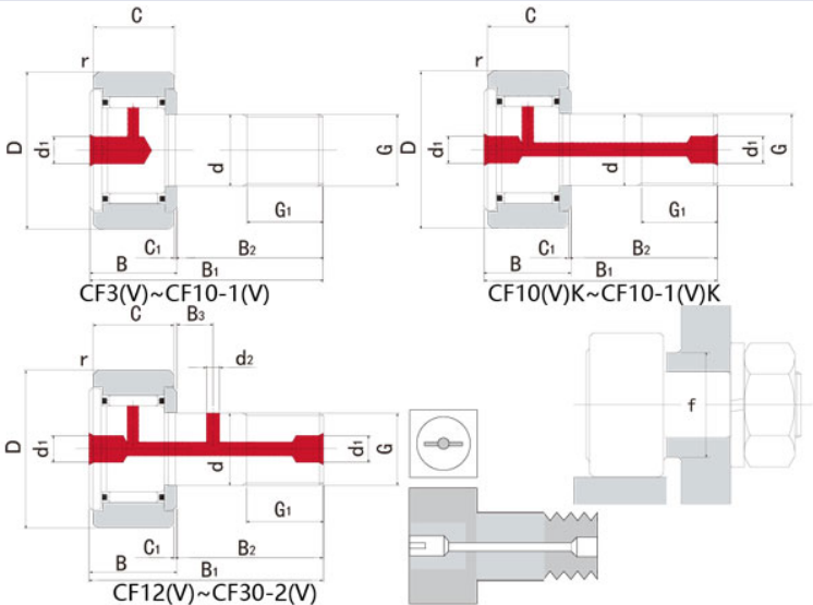
参数图
