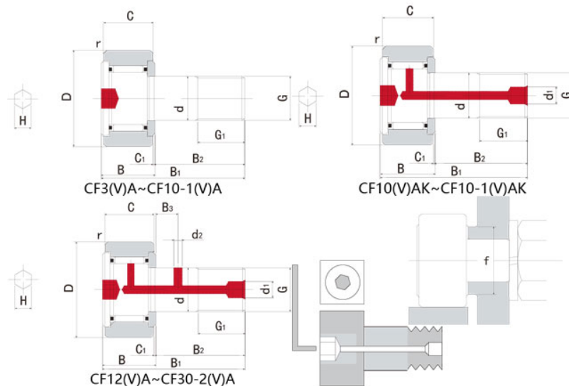
参数图
